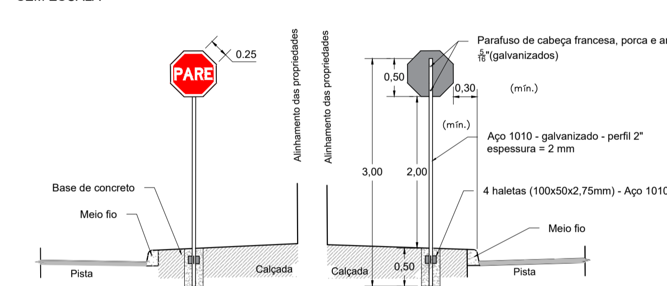
PLACA DE REGULAMENTAÇÃO OCTOGONAL SEM ESCALA
