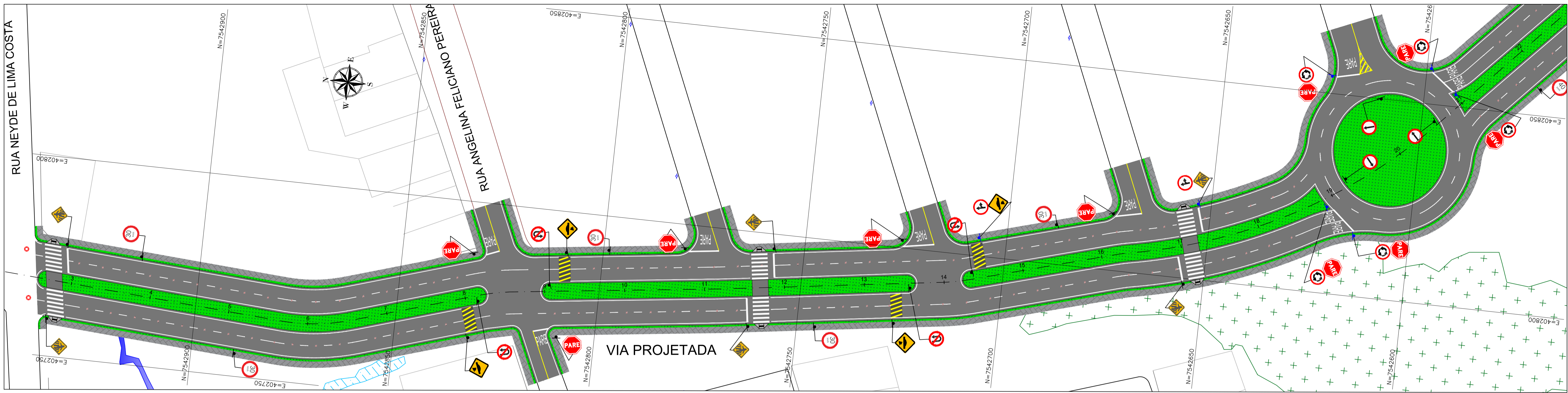
LINHA DE BORDO E TACHAS - LBO SEM ESCALA
