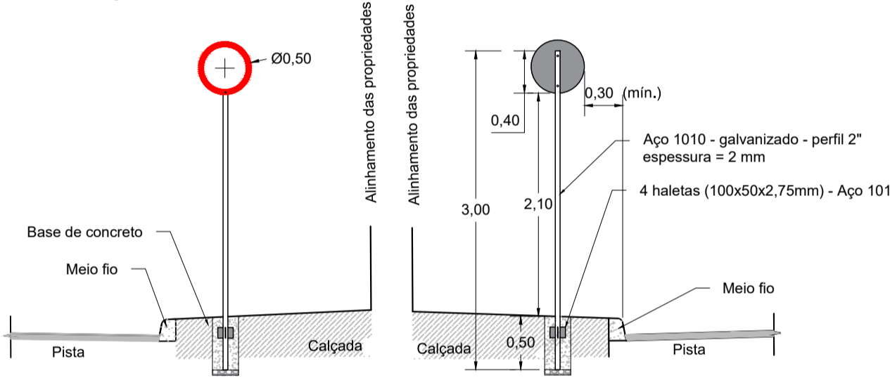
PLACA DE REG. CIRCULAR SEM ESCALA
