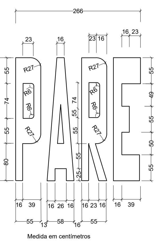
LEGENDA DE PARE SEM ESCALA
