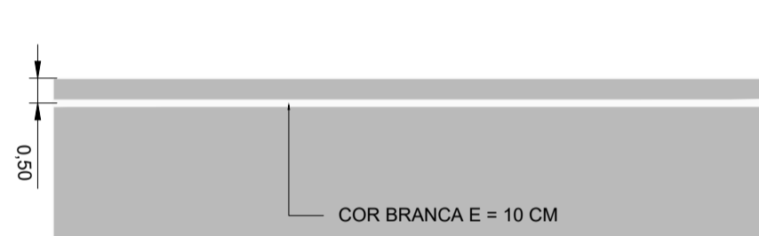
LINHA DE BORDO E TACHAS - LBO SEM ESCALA
