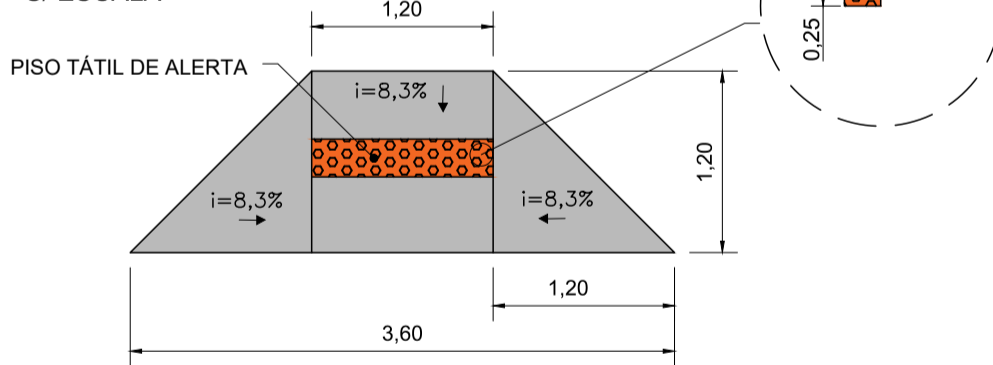
DETALHE - REBAIXO ACESSIBILIDADE TIPO 1 S/ ESCALA
