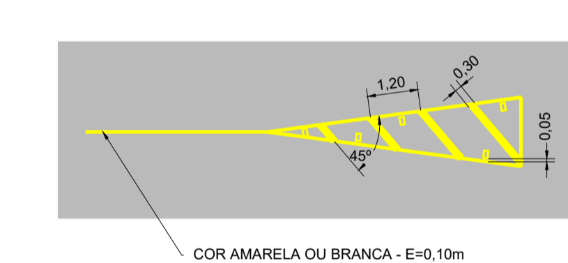
DETALHE - DISPOSITIVO AUXILIAR DELIMITADOR SEM ESCALA
