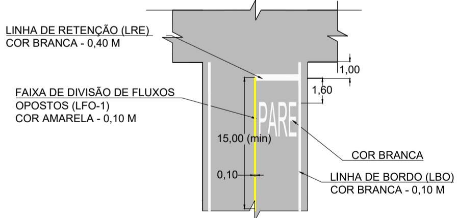
DETALHE - PINTURA SINALIZAÇÃO: PARADA OBRIGATORIA SEM ESCALA
