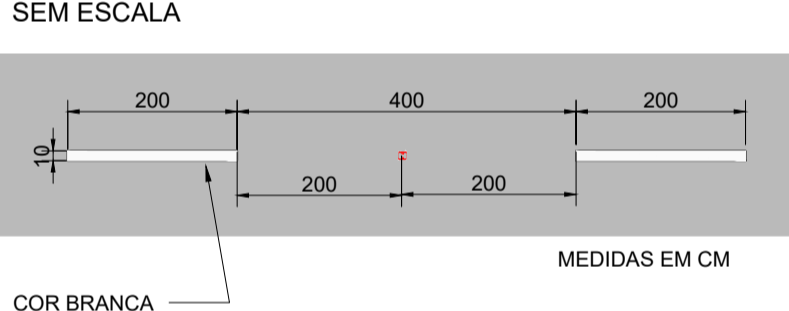
LINHA SIMPLES SECCIONADA LMS-2 SEM ESCALA
