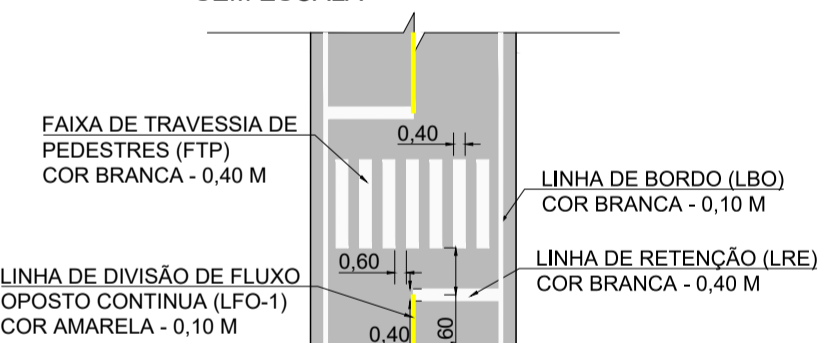
DETALHE C - FAIXA DE PEDESTRE SEM ESCALA
