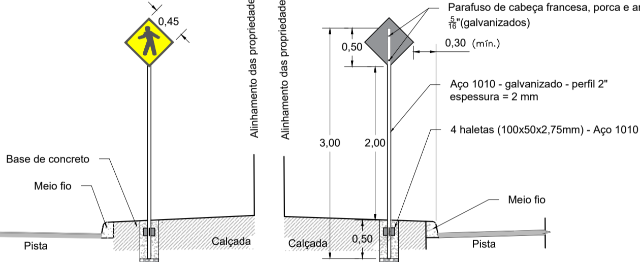
PLACA DE ADVERTÊNCIA SEM ESCALA
