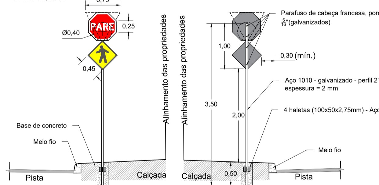
PLACA DE ADVERTÊNCIA E REG SEM ESCALA
