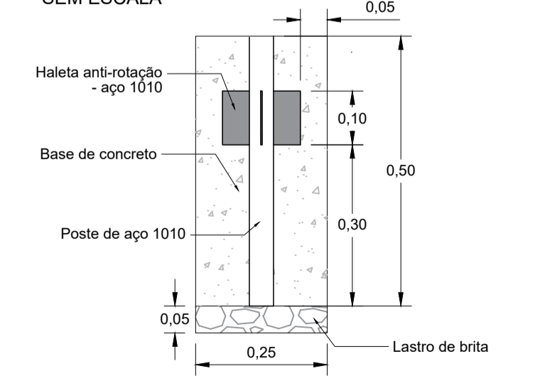
DET. DE FIXAÇÃO DE POSTES PARA PLACAS SEM ESCALA
